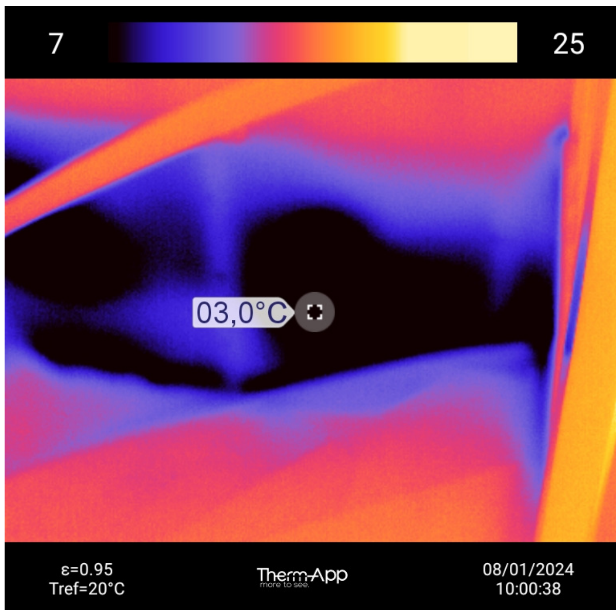
Knevegg i trappeåpning, kaldt område i knevegg langs etasjeskillet
